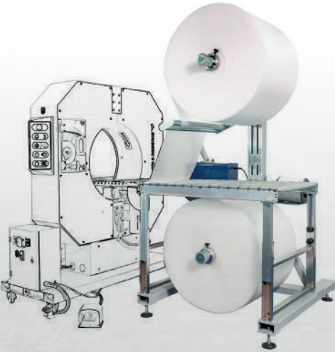
COMPATIBILE CON LE AVVOLGITRICI ORIZZONTALI MANUALI COMPACTA, NUOVE O GIÀ INSTALLATE. COMPATIBLE WITH MANUAL HORIZONTAL WRAPPING MACHINES COMPACTA, NEW OR ALREADY INSTALLED.
