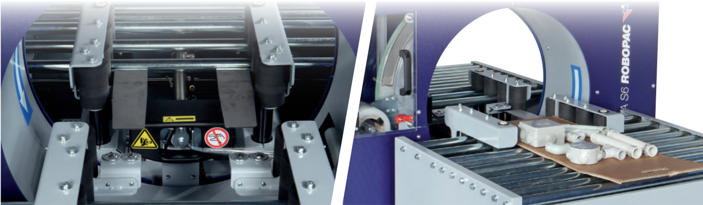
CONVOGLIATORE A RULLI VERTICALI MOTORIZZATI, REGOLABILI MANUALMENTE IN LARGHEZZA E DETTAGLIO GRUPPO PINZA E TAGLIO. VERTICAL MOTORIZED ROLLERS CONVEYORS, MANUAL WIDTH ADJUSTABLE/ CLAMPING-CUTTING DETAIL.
