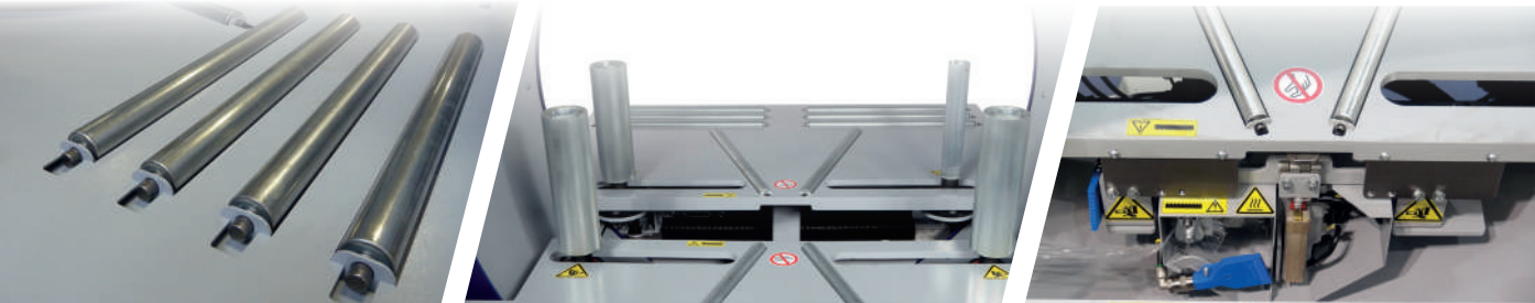
CONVOGLIATORE A RULLI (entrata+uscita) ROLLERS CONVEYOR (in+out) GUIDE AUTOCENTRANTI PNEUMATICHE E MOTORIZZATE / PNEUMATIC AND MOTORIZED SELF CENTERING GUIDES GRUPPO PINZA, TAGLIO (saldatore opz.) CLAMPING-CUTTING SYSTEM (welder opt.)
